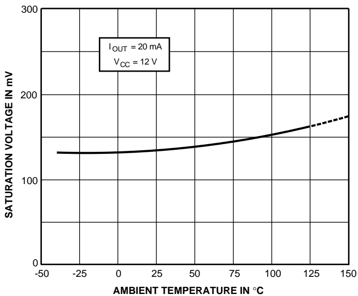
Dwg. GH-029-1
