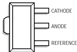
SOT-89 (S)
