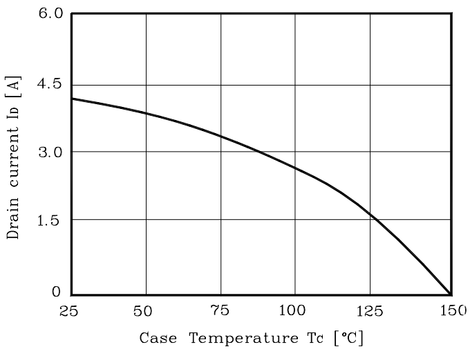
Fig. 9 I_D - T_C
