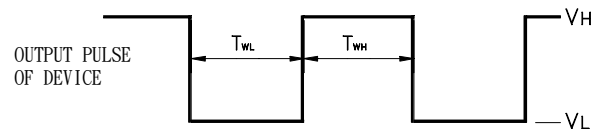
D.U.T output Pulse
